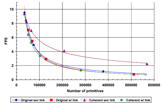
Figure 7: Images par seconde obtenues via notre approche par rapport au nombre de tétraèdres affichés via un DVR.
